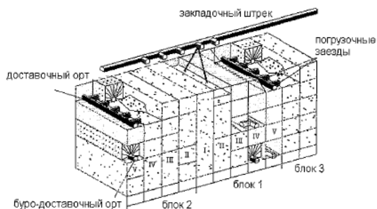
Рисунок 1 – Схема обработки блока подэтажно-камерной системой разработки со сплошной выемкой руды и закладкой.
