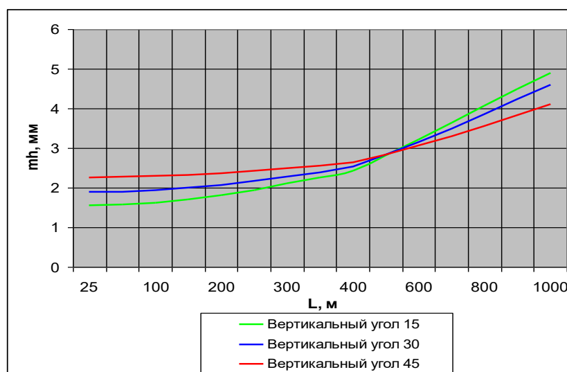
Сурет 1. Тік бұрыштың арақашықтықты ұлғайта отырып, репердің биіктік белгісін анықтау дәлдігіне әсері
