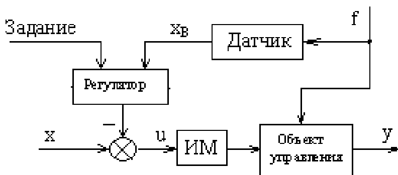
Рисунок 1 - Структурная диаграмма неисправности САУ
