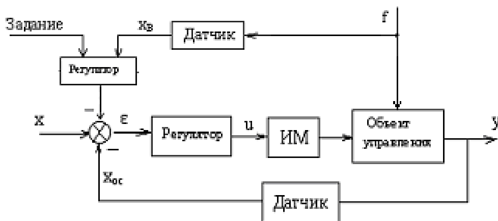
Рисунок 2 - Блок-схема комбинированной САУ
