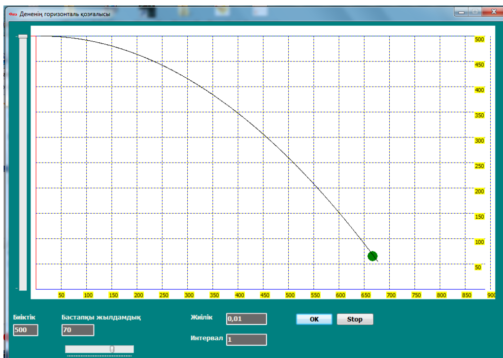
2-сурет. Горизонталь лақтырылған дене қозғалысы.
