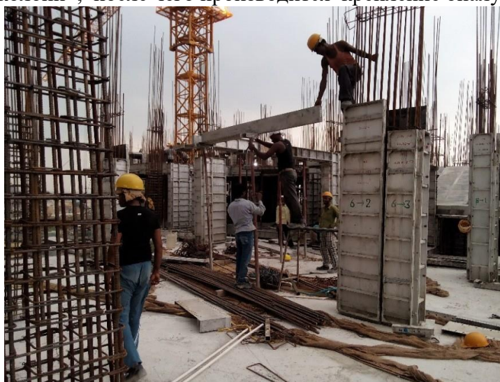
Рисунок 3. Показано крепление “Миванной” плиты на колонне.
